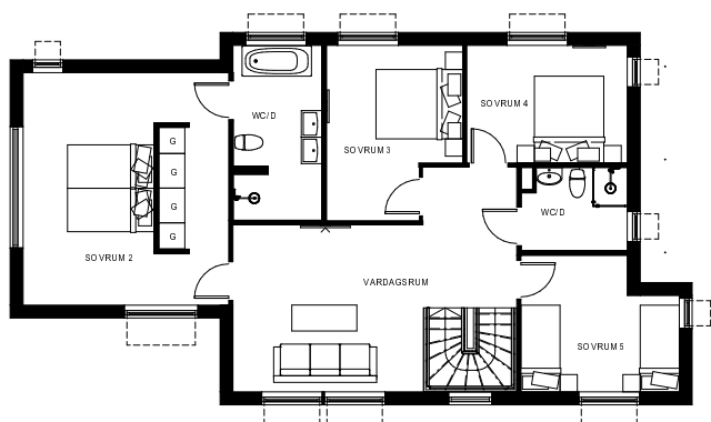
ÖVERVÅNING 101 KVM
